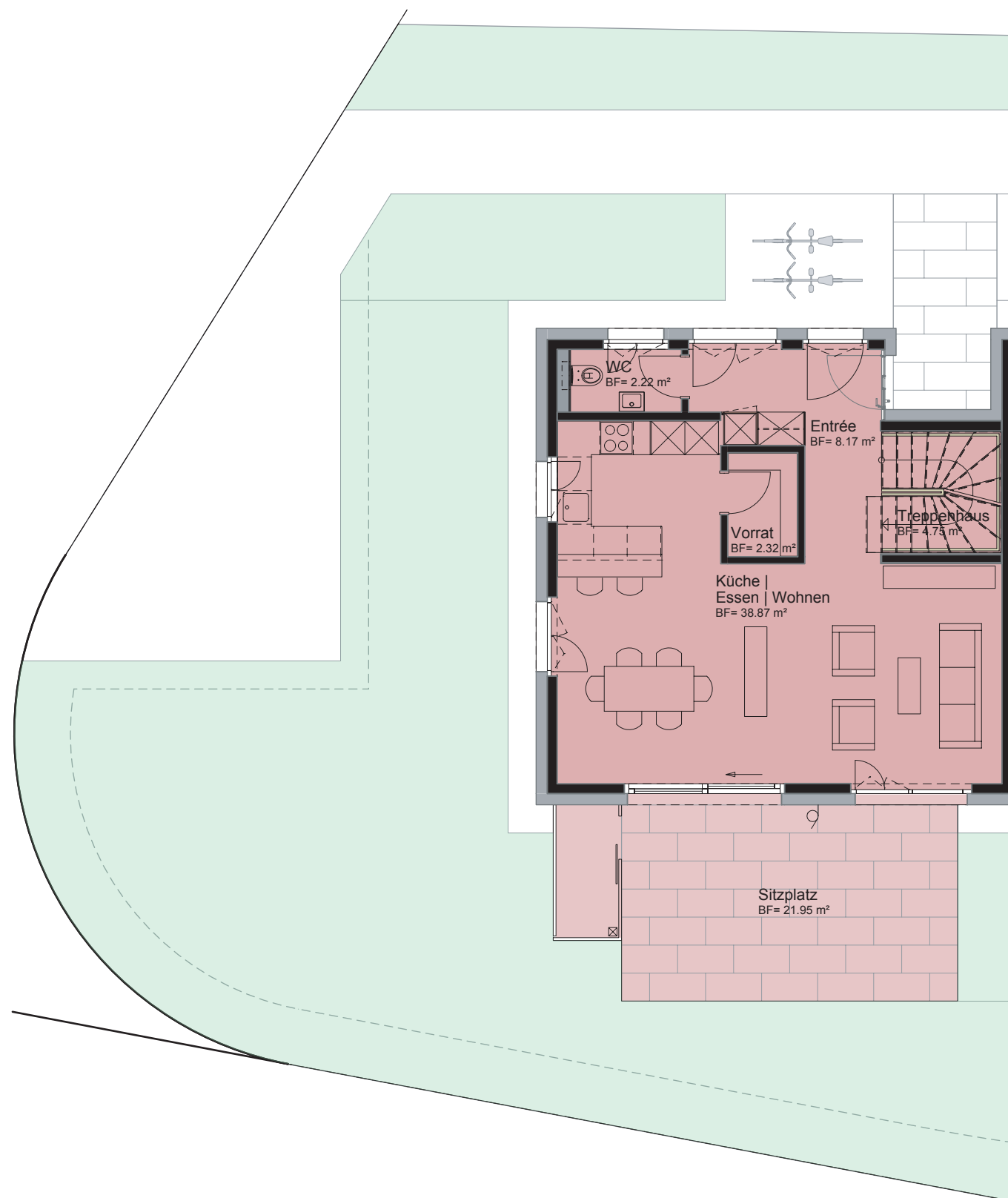
ERDGESCHOSS
