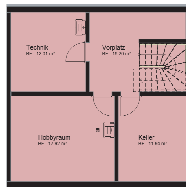
UNTERGESCHOSS
