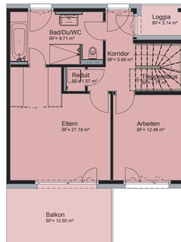
OBERGESCHOSS
