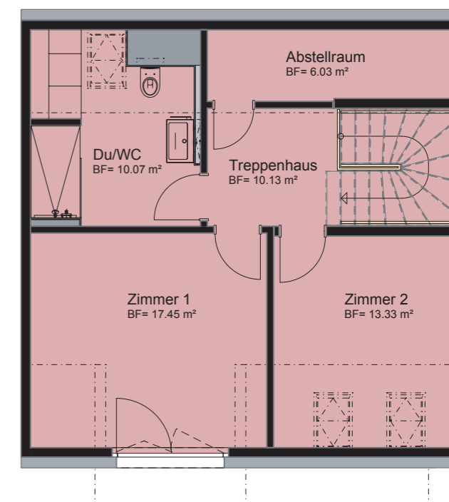
DACHGESCHOSS
